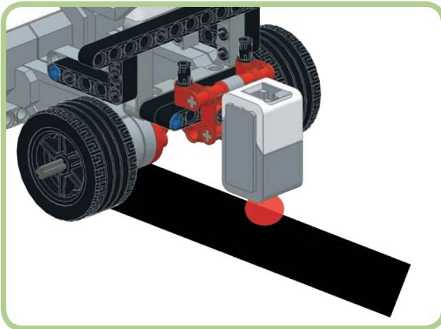
Abbildung 6-5: Der Farbsensor über dem Rand der Linie
