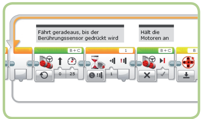
Abbildung 6-22: Das Programm BumperBot2
