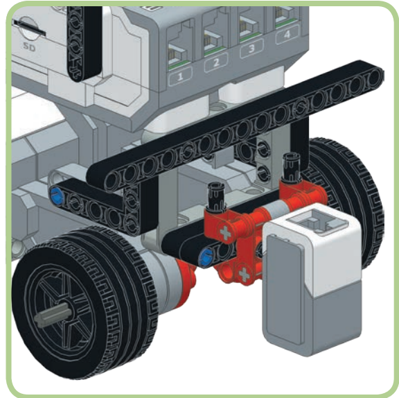
Abbildung 6-3: Der Farbsensor in der Stellung zum Verfolgen einer Linie
