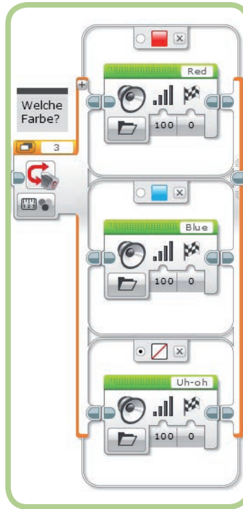
Abbildung 6-16: Keine Farbe als Standardfall
