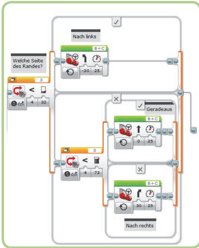
Abbildung 6-9: Die Schwellenwerte festlegen
