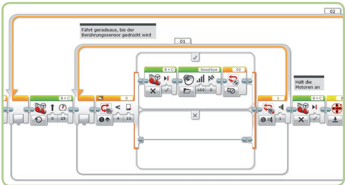
Abbildung 6-23: Das Programm BumperBot3
