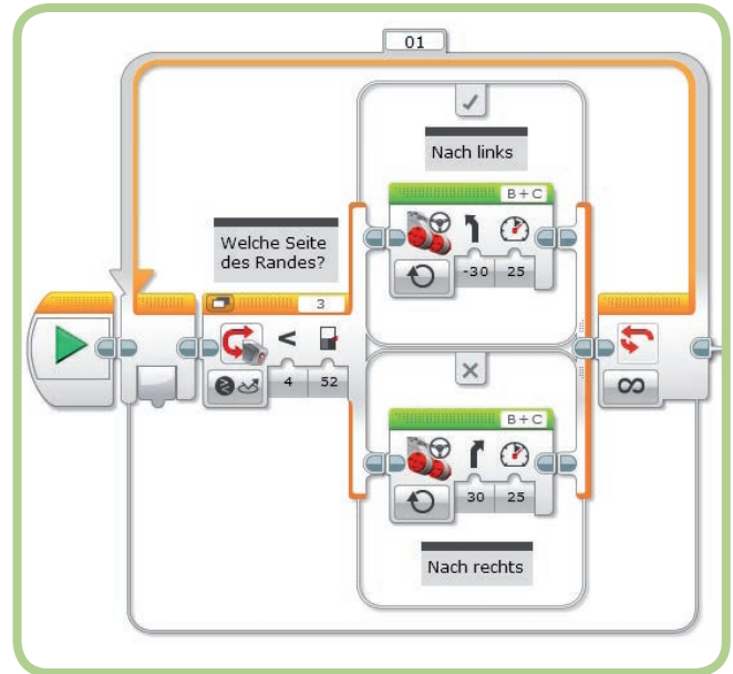
Abbildung 6-6: Das Programm LineFollower
