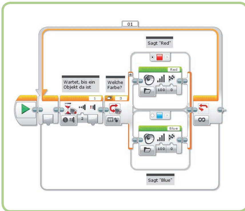
Abbildung 6-13: Rote und blaue Objekte identifizieren
