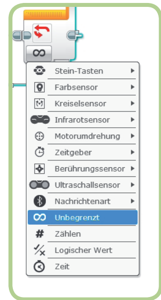
Abbildung 6-17: Den Modus eines Schleifenblocks auswählen
