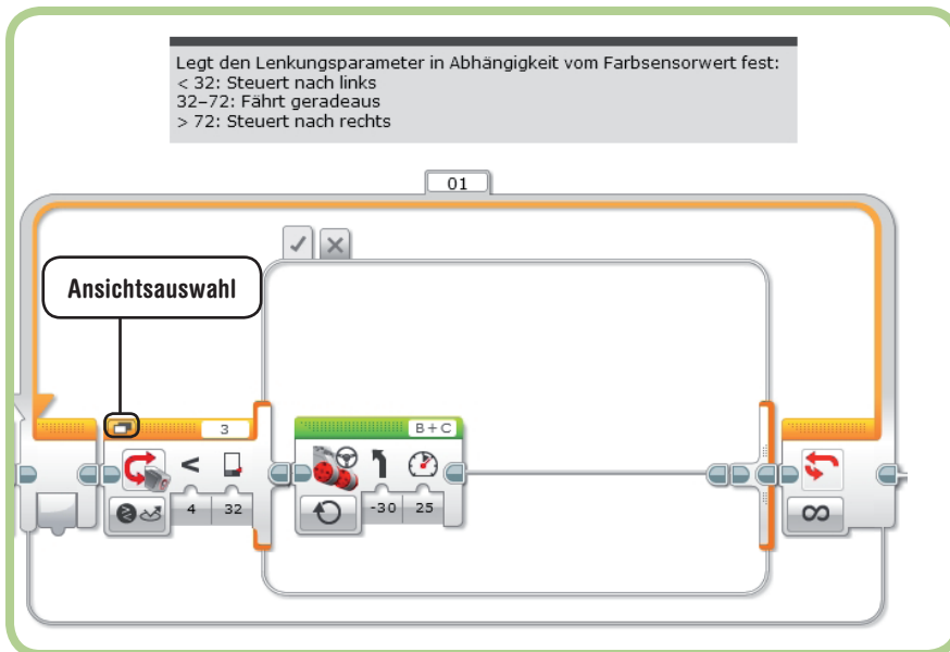
Abbildung 6-10: Der Schalterblock in der Registeransicht
