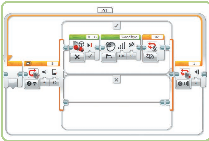
Abbildung 6-26: Die Motoren anhalten und »Goodbye« sagen
