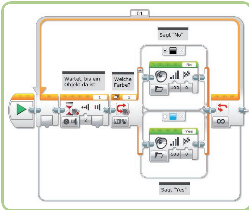
Abbildung 6-11: Der Ausgangspunkt für das Programm RedOrBlue
