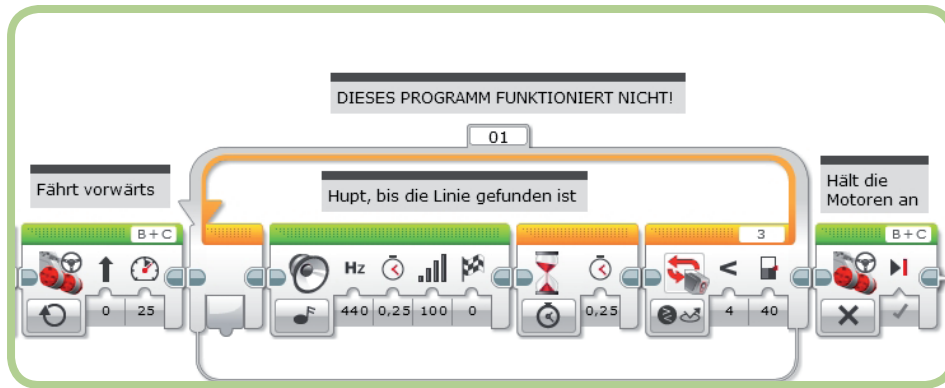
Abbildung 6-18: Eine fehlerhafte Version des Programms LineFinder
