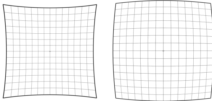
Abb. 3.48 Links: die kissenförmige Verzeichnung (die Linien des Motivs biegen sich zu den Rändern hin nach außen); rechts: die tonnenförmige Verzeichnung (Linien biegen sich zu den Rändern hin nach innen)
