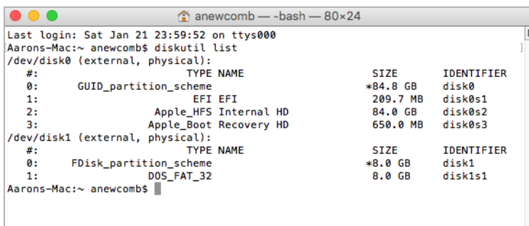
Abb. 1-7 Beispiel einer Ausgabe nach dem Befehl diskutil list
