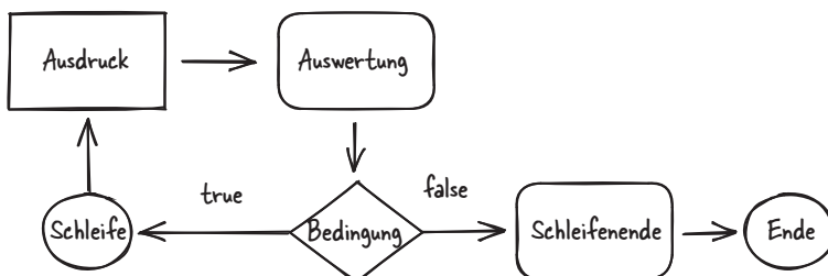
Abbildung 2-3: Logik einer do while -Schleife
