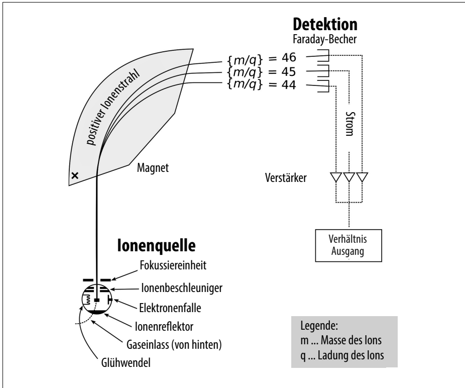
Abbildung 4-1: Schematische Skizze eines Massenspektrometers. (Quelle: Wikimedia, https://commons.wikimedia.org/wiki/File:Mass_Spectrometer_Schematic.svg )
