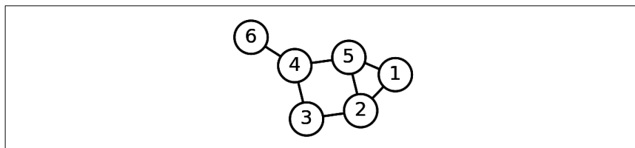
Abbildung 4-5: Beispiel eines mathematischen Graphen mit sechs Knoten, der durch Kanten verbunden wird. (Quelle: Wikimedia, https://commons.wikimedia.org/wiki/File:6n-graf.svg )
