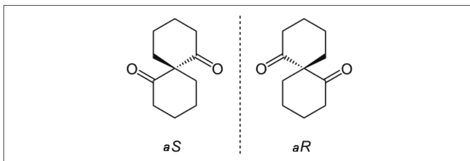
Abbildung 4-9: Axiale Chiralität einer Spiroverbindung (einer Verbindung aus zwei oder mehr miteinander verbundenen Ringen). Beachten Sie, dass die beiden chiralen Varianten jeweils mit »R« und »S« gekennzeichnet sind. Diese Konvention ist in der chemischen Literatur sehr verbreitet.
