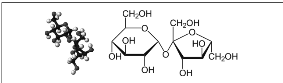
Abbildung 4-7: Saccharose, dargestellt als 3-D-Konformation und chemische 2-D-Struktur. Bilder aus Wikimedia ( https://commons.wikimedia.org/wiki/File:Sucrose-3D-balls.png ) und Wikipedia ( https://en.wikipedia.org/wiki/File:Saccharose2.svg ).
