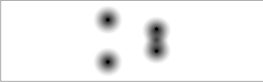
Abbildung 4-3: Links: zwei Atomkerne, jeder umgeben von einer Elektronenwolke. Rechts: Nähern die Atome sich an, verbringen die Elektronen mehr Zeit im Raum zwischen den Kernen. Dies zieht die Kerne zusammen und bildet eine kovalente Bindung zwischen den Atomen.
