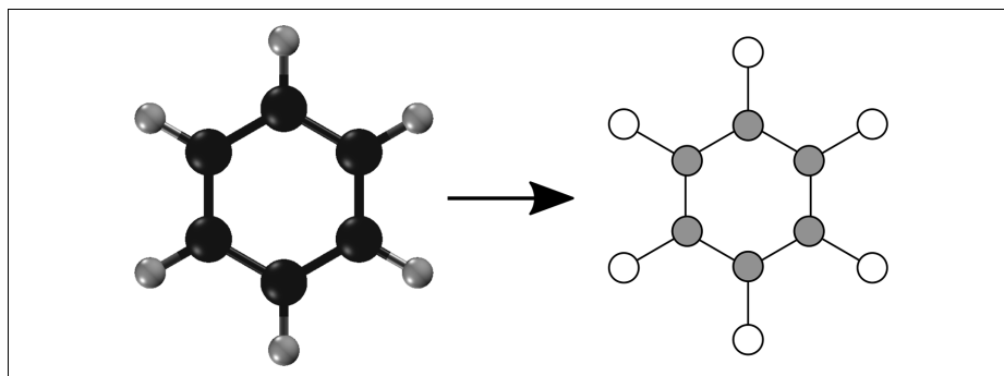
Abbildung 4-6: Ein Beispiel für die Umwandlung eines Benzolmoleküls in einen Molekülgraphen. Beachten Sie, dass Atome in Knoten und chemische Bindungen in Kanten umgewandelt werden.
