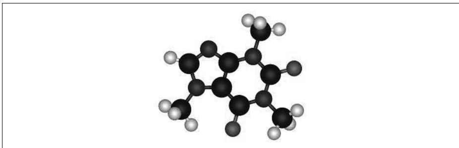
Abbildung 4-2: Eine einfache Darstellung eines Koffeinmoleküls als Kugel-Stab-Modell. Atome werden als farbige Kugeln dargestellt (Schwarz für Kohlenstoff, Rot für Sauerstoff, Blau für Stickstoff, Weiß für Wasserstoff), die mit Stäbchen verbunden sind, die chemische Bindungen symbolisieren.
