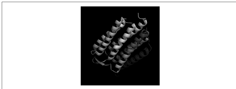
Abbildung 4-8: Eine in 3-D gerenderte Konformation von Bacteriorhodopsin (zur Erfassung von Lichtenergie). Proteinkonformationen sind besonders komplex und enthalten mehrere geometrische 3-D-Motive. Sie erinnern daran, dass Moleküle zusätzlich zu ihren chemischen Formeln auch eine Geometrie aufweisen. (Quelle: Wikimedia, https://upload.wikimedia.org/wikipedia/commons/thumb/d/dd/1M0K.png/480px-1M0K.png )
