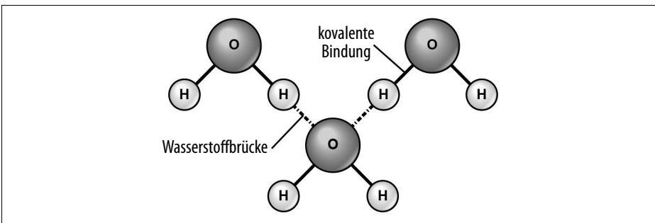
Abbildung 4-4: Wassermoleküle bilden starke Wasserstoffbrücken zwischen Wasserstoff und Sauerstoff an benachbarten Molekülen aus. Ein solides Netzwerk von Wasserstoffbrücken trägt zum Teil zur Stärke des Wassers als Lösungsmittel bei. (Quelle: Wikimedia, https://commons.wikimedia.org/wiki/File:SimpleBayesNet.svg )
