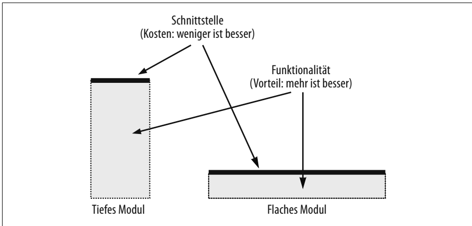
Abbildung 4-1: Tiefe und flache Module. Die besten Module sind tief: Sie erlauben, viel Funktionalität über eine einfache Schnittstelle anzusprechen. Ein flaches Modul ist eines mit einer recht komplexen Schnittstelle, aber nicht viel Funktionalität – so wird nicht viel Komplexität verborgen.
