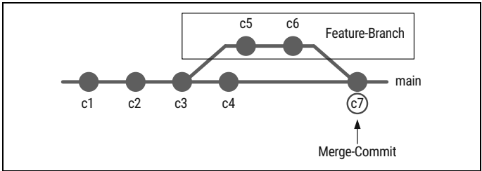
Abbildung 3-10: Gab es Änderungen im main -Branch, führt Git einen 3-Wege-Merge durch und erstellt einen Merge-Commit.
