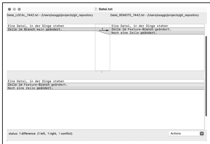
Abbildung 3-11: Ein Screenshot des Merge-Tools FileMerge
