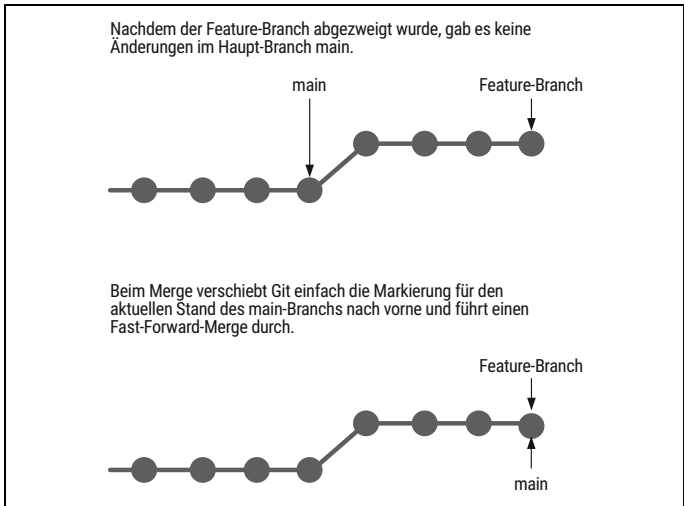
Abbildung 3-9: Ein Fast-Forward-Merge in Git
