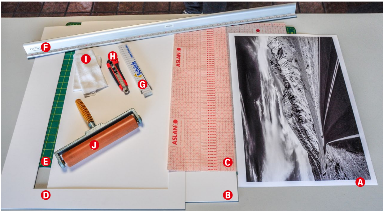
[1] Material (Druck, Rückenkarton, Klebefolie, Passepartout) sowie Werkzeuge (Schneidematte, Schneidelineal, Maßstab, Messer, Tuch oder Walze) für das Aufziehen von Bildern
