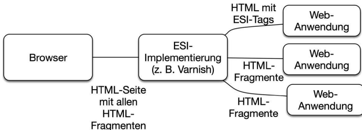
Abb. 1 ESI-Konzept: HTML-Fragmente zu HTML-Seiten integrieren
