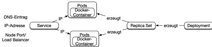
Abb. 4 Zusammenspiel der Kubernetes-Konzepte
