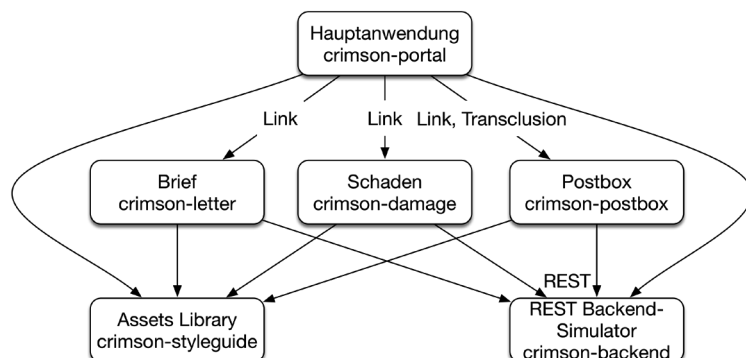
Abb. 2 Integration mit Links und JavaScript
