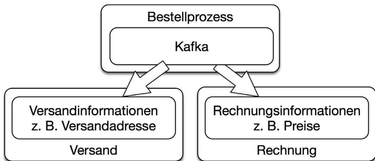
Abb. 3 Überblick über das Kafka-Beispiel
